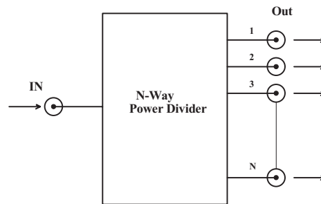
Fig. 7 1 : N Power Divider/Coupler
